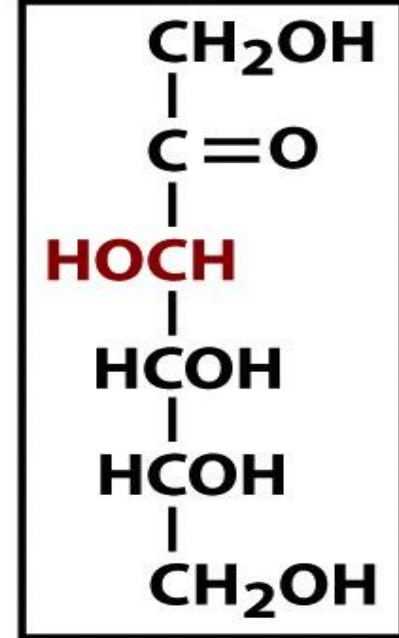
D-Fructose
